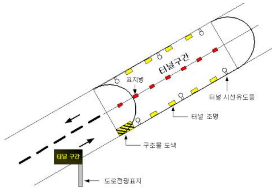
<그림 13> 터널의 시설 설치 예(양방향通行)
