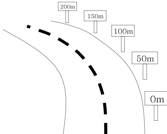
〈그림 6〉 안개 시정표지의 설치 형상
