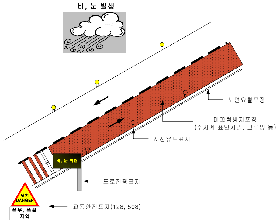
<그림 10> 비, 눈 등으로 인한 위험구간의 시설 설치 예(직선부)
