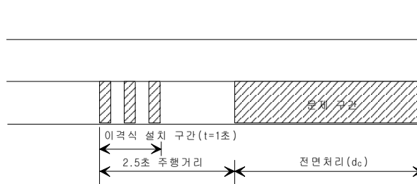
〈그림 2〉 미끄럼방지포장(수지계 표면처리) 설치 예
