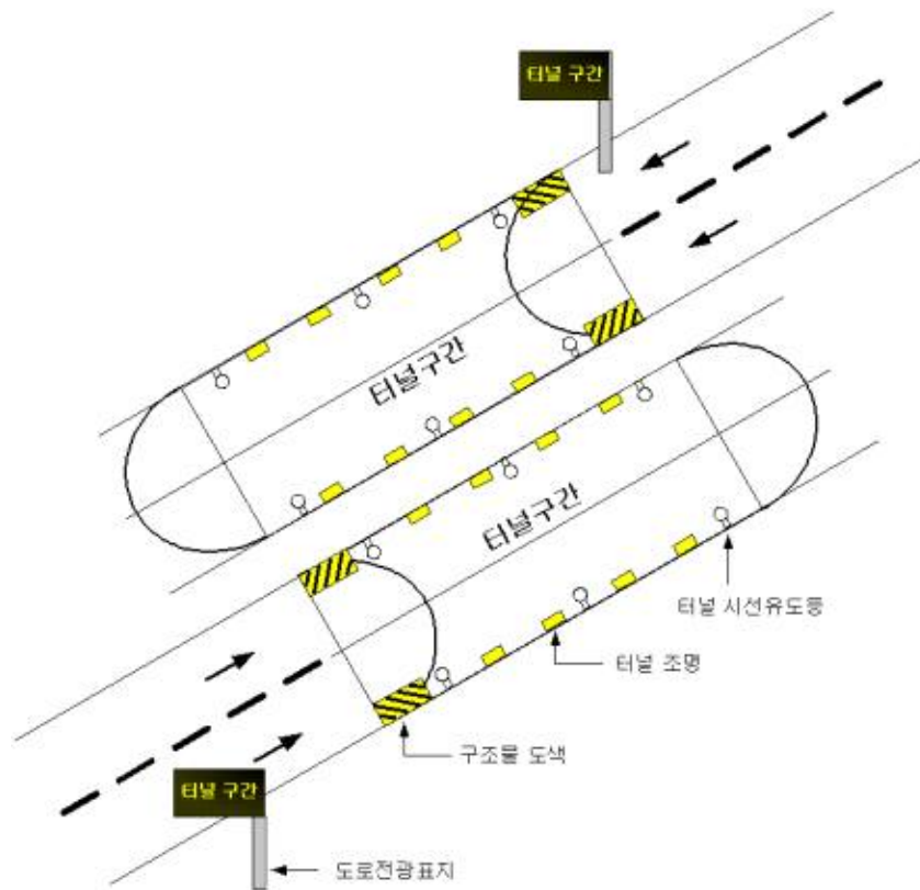
<그림 14> 터널의 시설 설치 예(일방향通行)
