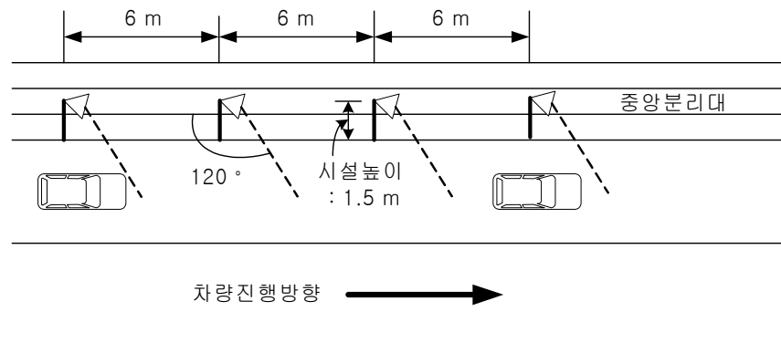
부록-그림 1.3 낮은 조명의 설치 제원(일본)
